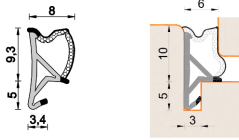
A 571 STP BOB Per serramenti in legno
