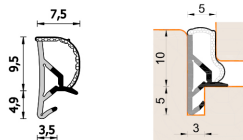
A 401 STP BOB Per serramenti in legno
