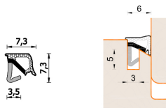
A 273 ESP BOB Per serramenti in legno
