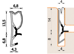
A 268 ESP BOB Per serramenti in legno
